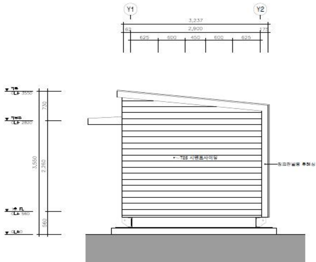
⑦ 좌측면도
