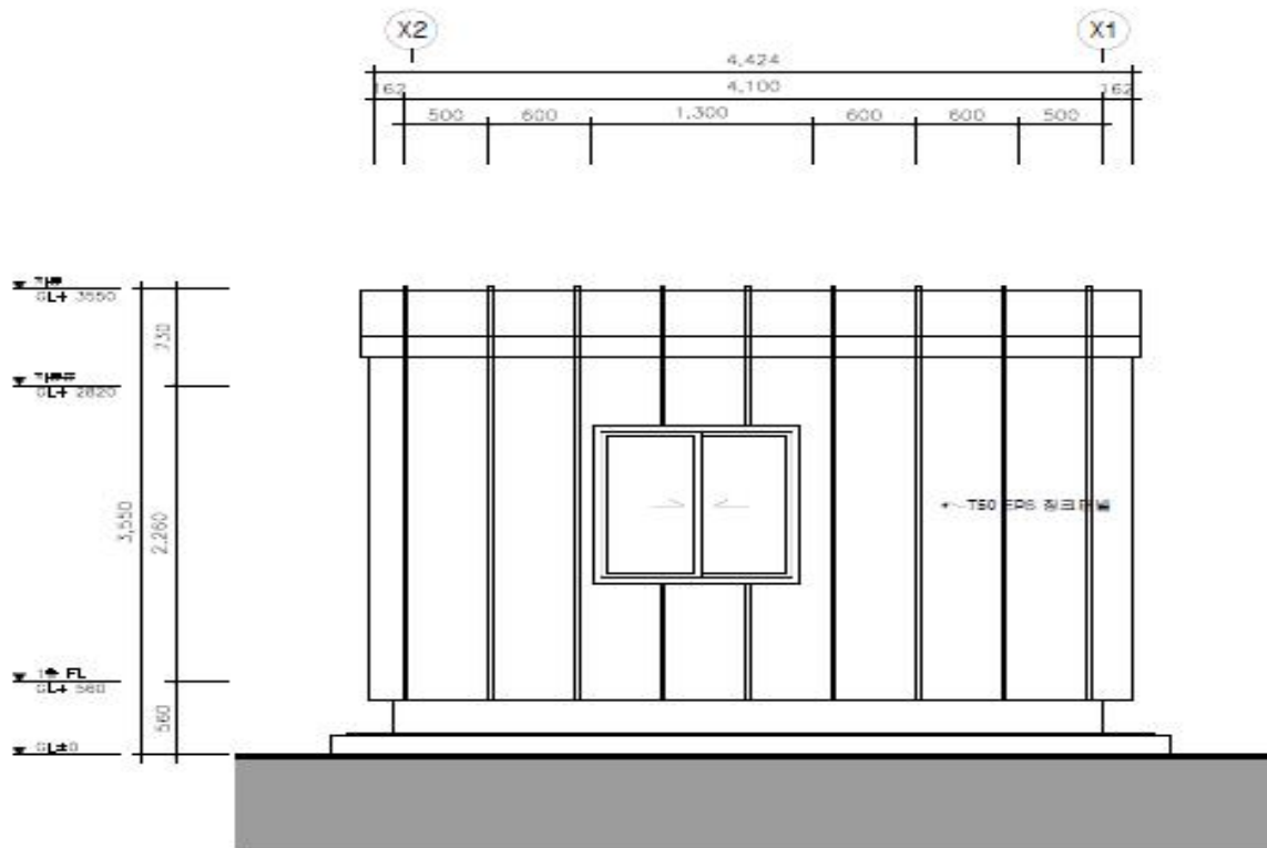
⑥ 우측면도
