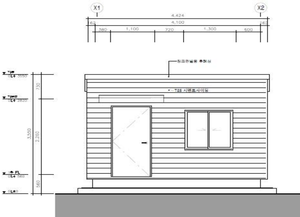
⑤ 배면도
