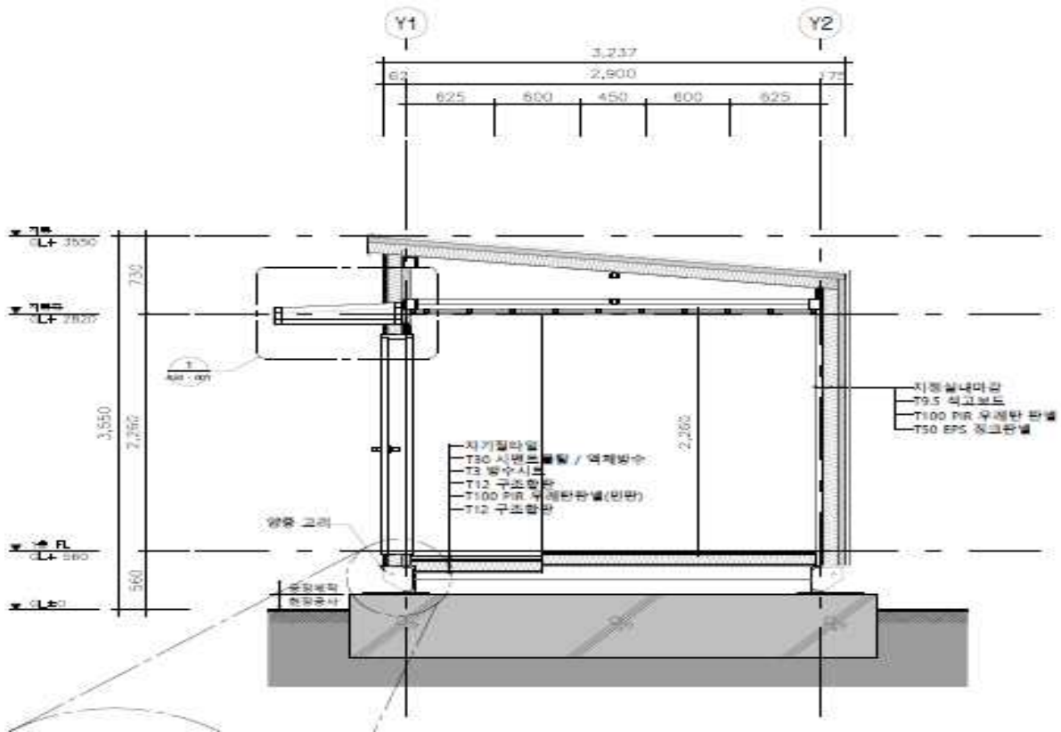
④ 정면도
